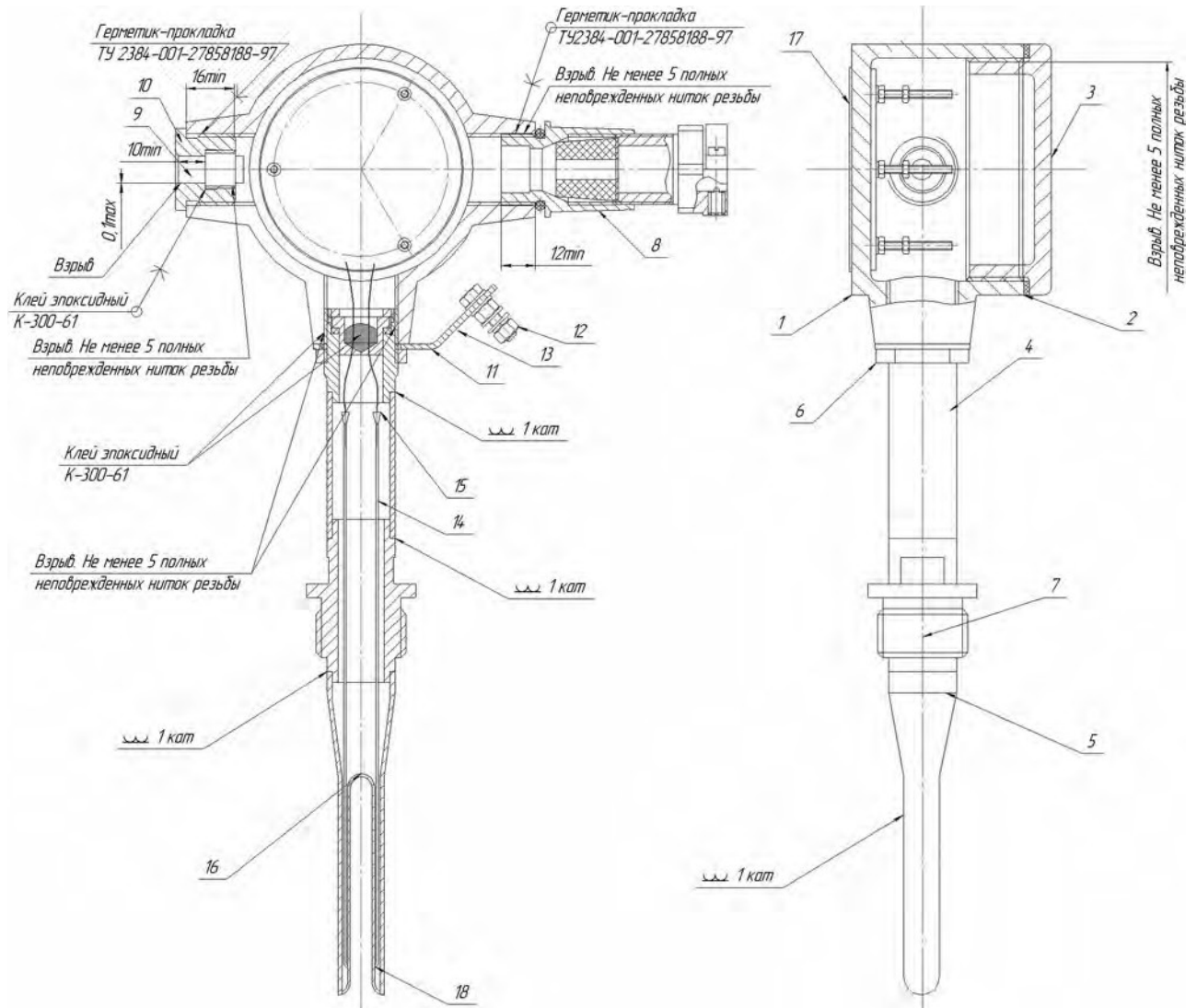
Рис.1А. Чертеж средств взрывозащиты прибора СЖУ-1-ОГ.
