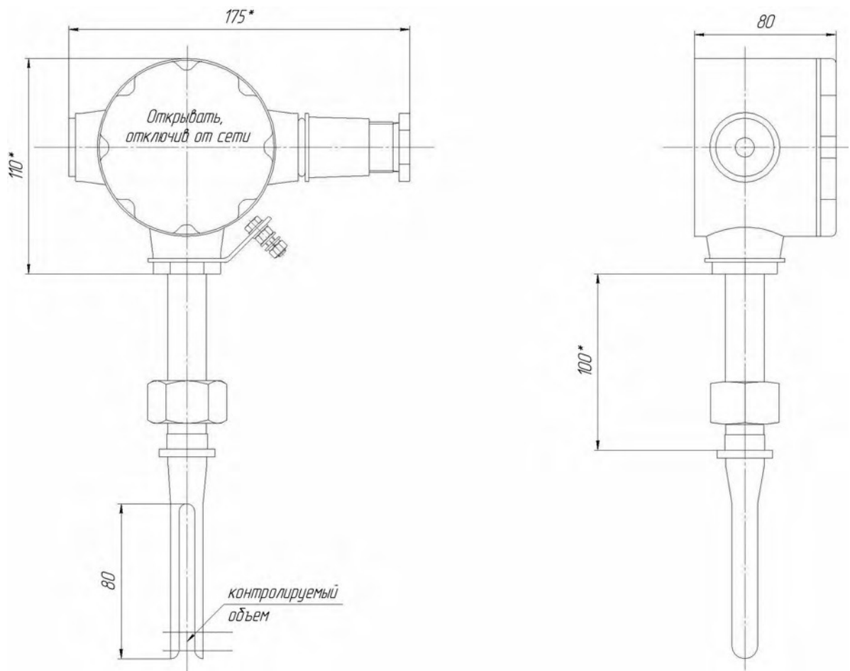
Рис. 1. Внешний вид прибора СЖУ-1-ОГ.
